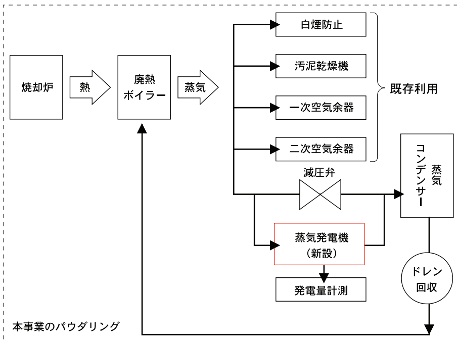
蒸気発電機設置フロー図
